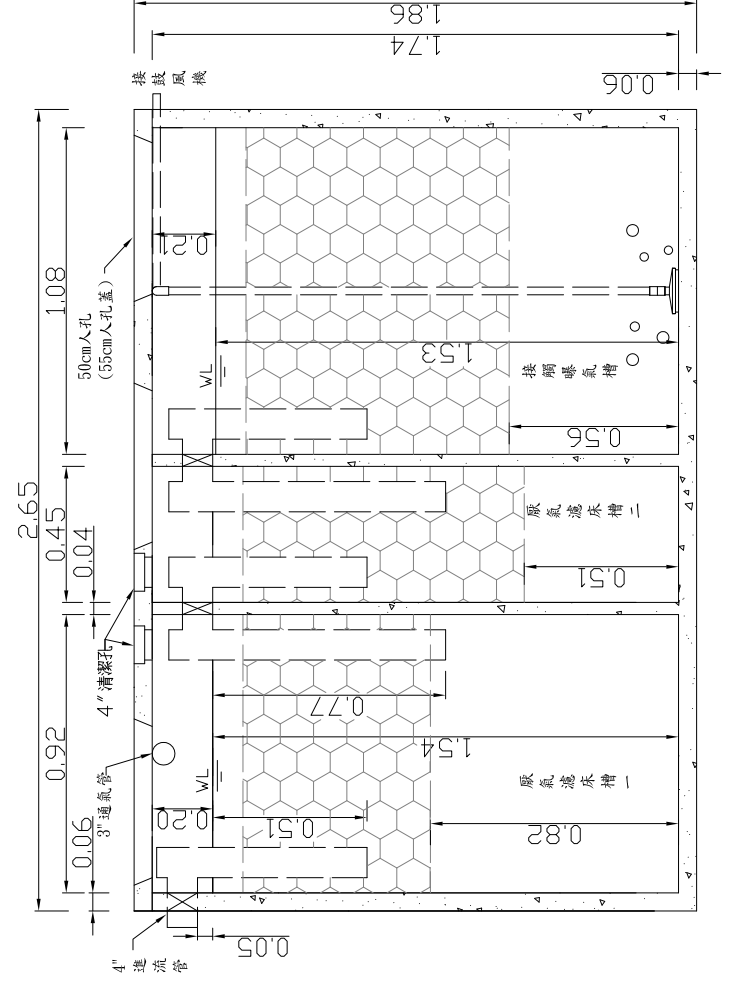
處理設施A-A剖面圖 單位:m 比例尺:1/25
